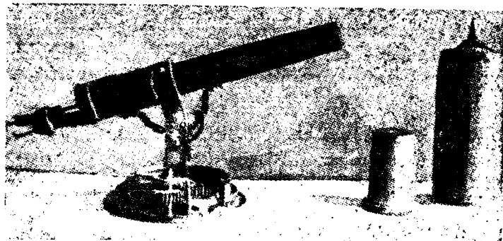
1. Пушка, изобретенная рабочим Сормовского завода Париковым. 2. Ручная бомба. 3. Фугасная бомба. Бомбы отливались в чугунолитейном и обрабатывались в механическом и инструментальном цехах Сормовского завода
